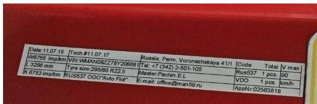
Фото 10. MAN.TGM-18.280-4X2-BB: идентификационная наклейка в дверном проеме транспортного средства.
