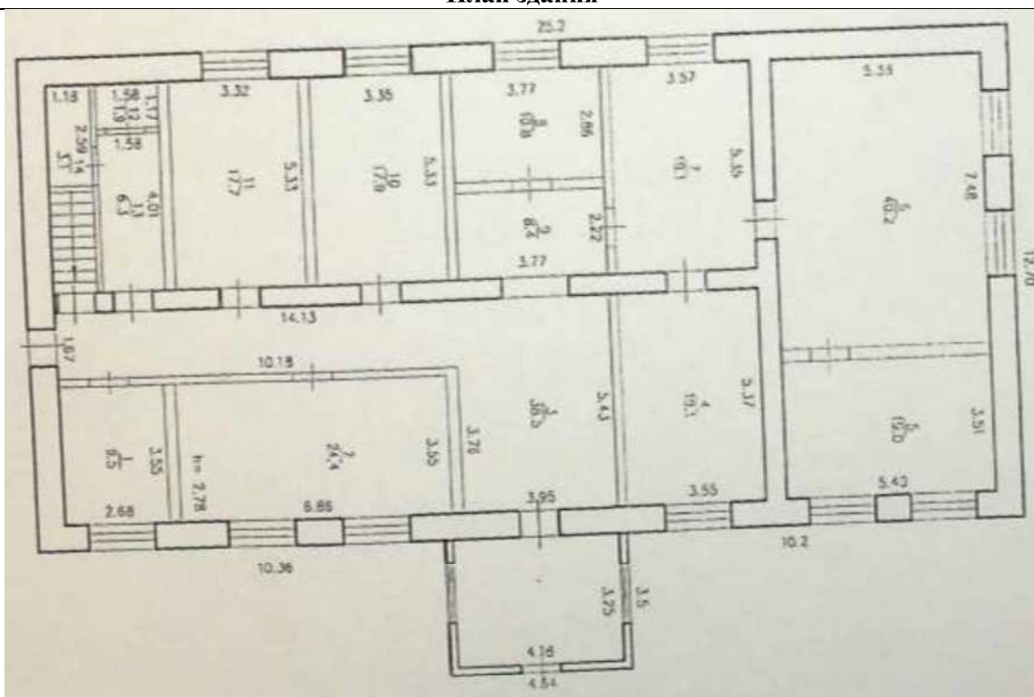
План здания
