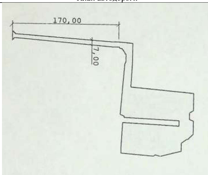
План автодороги
