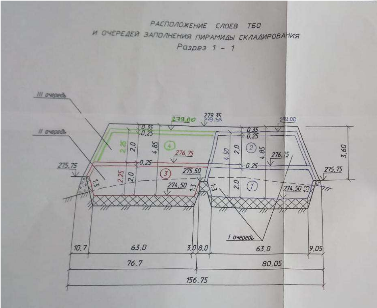
Поперечный профиль полигона
