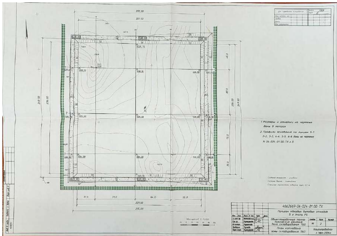
План котлована
