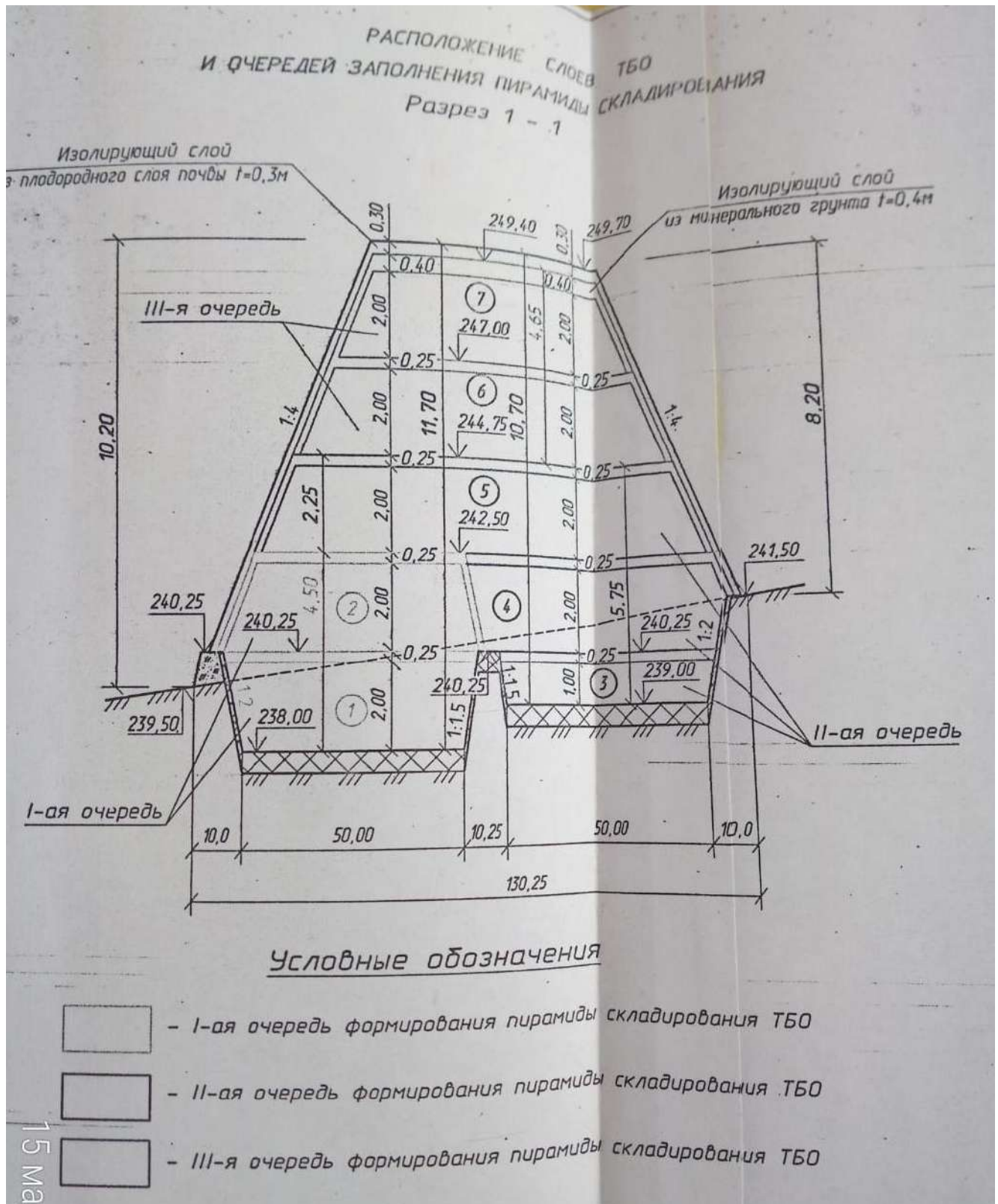
Поперечный разрез тела полигона (проект)
